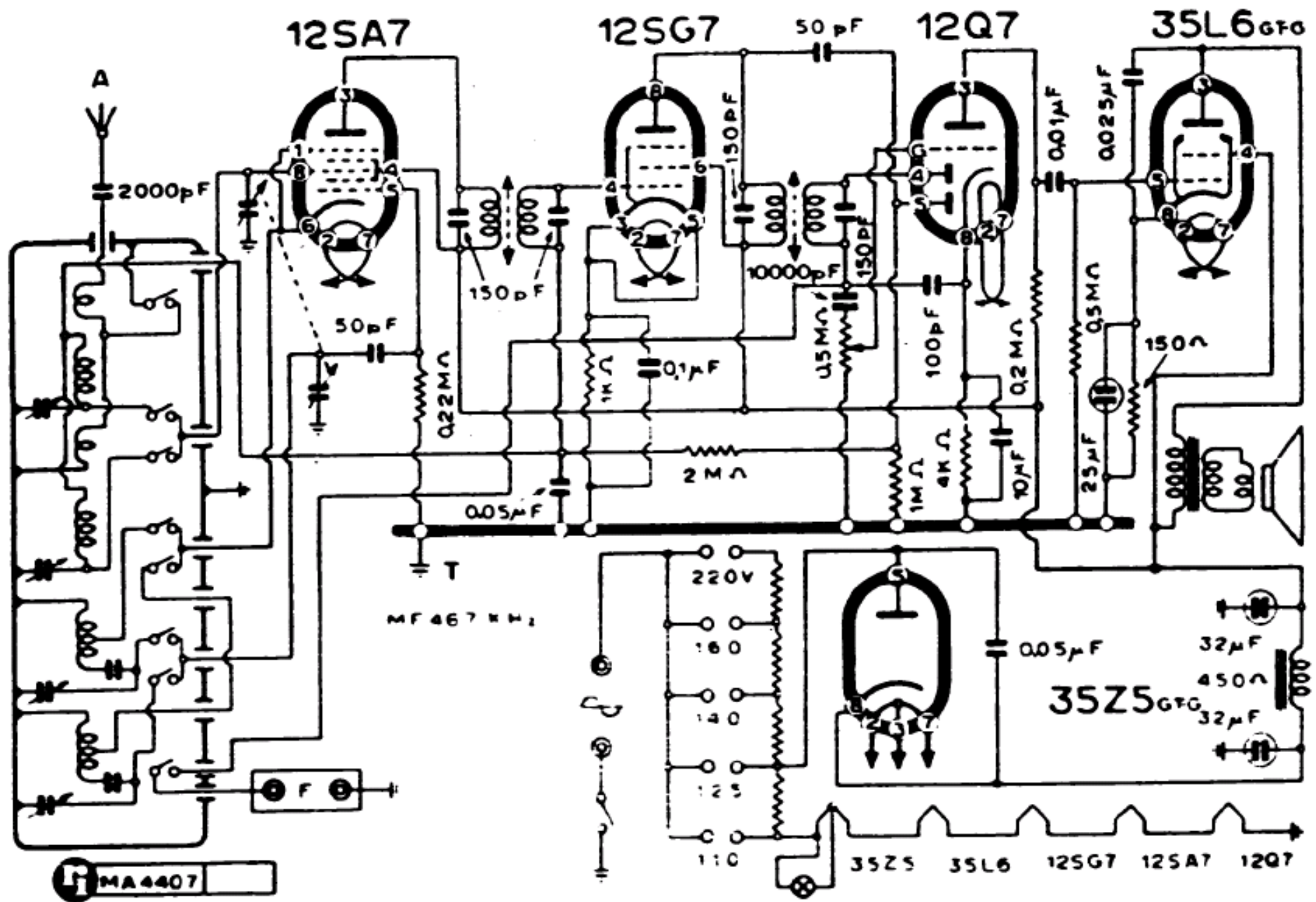
INCAR - MOD. « LV 56 »
